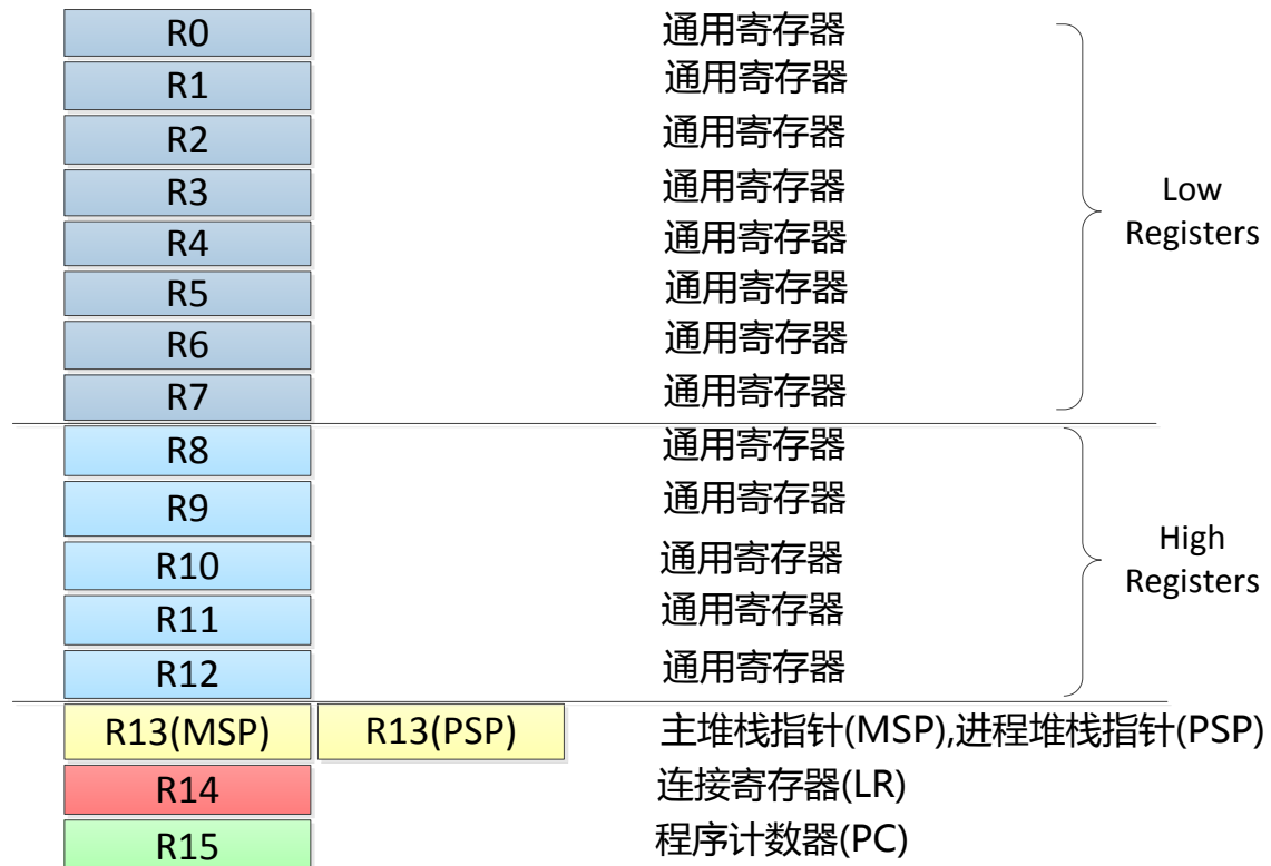
图 2.1.1 Cortex-M3/M4 通用寄存器
