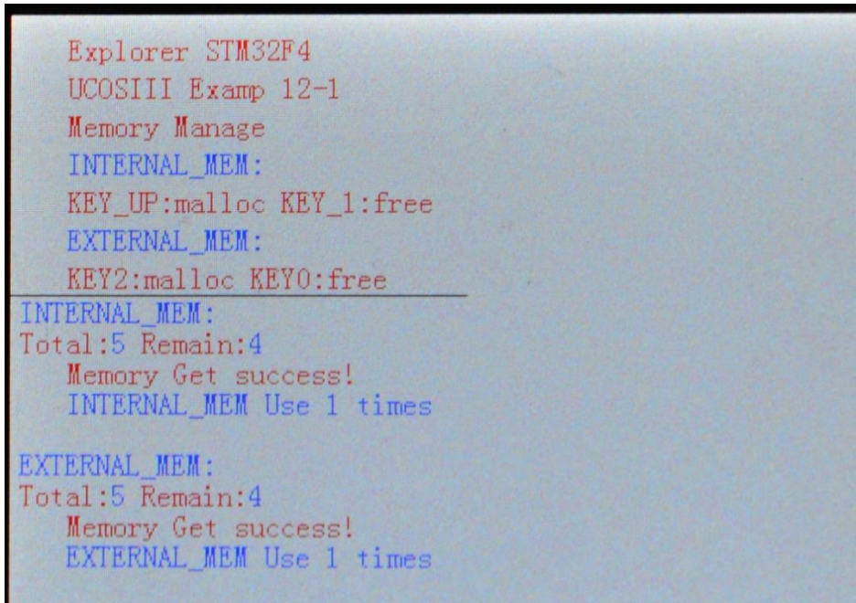
图 14.4.3 申请内存
