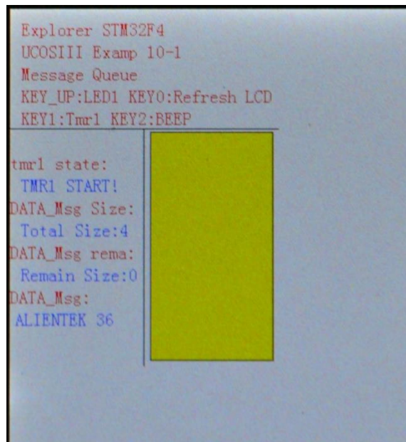
图 11.3.4 消息队列 DATA_Msg 剩余空间为 0
